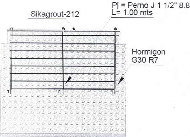
CORTE 2-2
