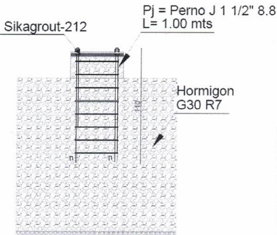
CORTE 1-1
